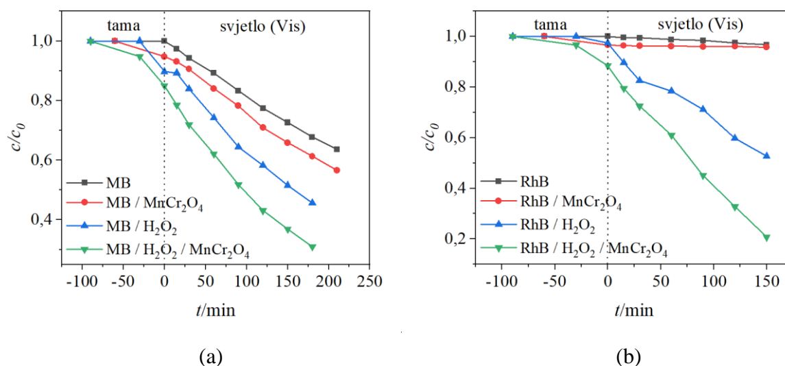
Slika 114. Učinkovitost razgradnje bojila (a) MB i (b) RhB nakon izlaganja vidljivom zračenju uz prisutnosti fotokatalizatora O4 i H 2 O 2 .
