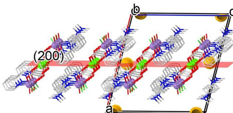
Slika 67. Žuta područja predstavljaju šupljine u koje se mogu smjestiti molecule vode u spoju 12 .
