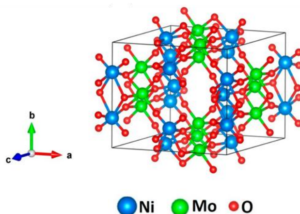
Slika 30. Kristalna struktura spoja \alpha -NiMoO 4 . 65
