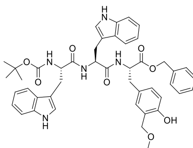
Shema 48. Priprava spoja 37
