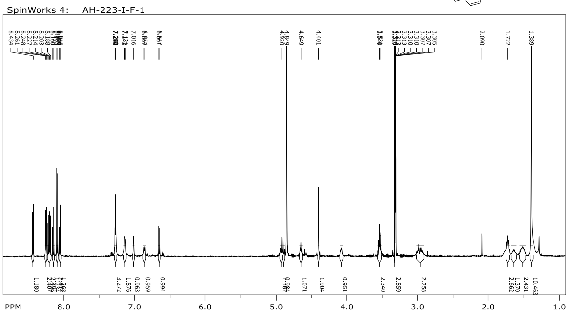
Prilog 81. ^{13}\text{C} NMR ( \text{CD}_3\text{OD} , 150 MHz) spektar Boc-Lys(Pyr)-Tyr[CH 2 OCH 3 ]-OBn ( 50 )
