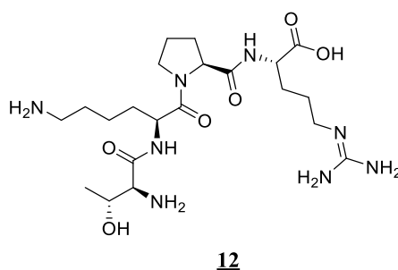
Slika 13. Struktura tuftsina
