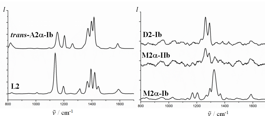
Slika 4.5: Raman spektri liganda L2 , izoliranog adukta A2α-Ib i izoliranih ciklopaladiranih spojeva M2α-Ib , M2α-IIb i D2-Ib .
