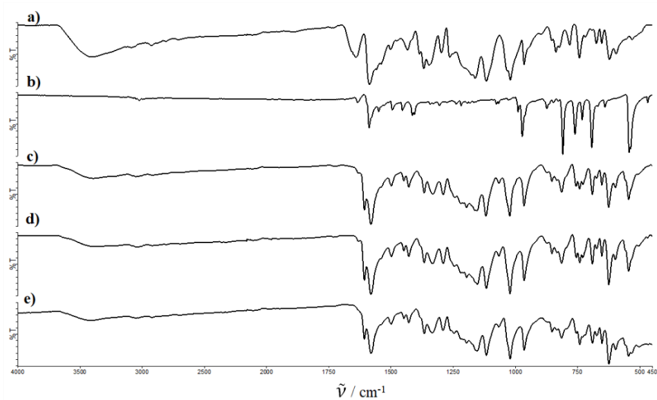
Slika 8.66: IR spektri: a) prekursora D2-Ib , b) 4-stirilpiridina, c) produkta D1-Ie , d) produkta ispranog vodom, e) produkta prekrizaliziranog iz MeOH.
