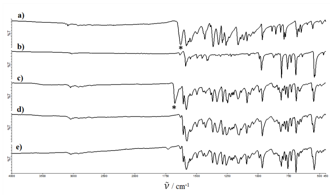
Slika 8.67: IR spektri: a) prekursora D3-Ib , b) 4-stirilpiridina c) produkta D3-Ie , d) produkta ispranog vodom, e) produkta prekrizaliziranog iz MeOH. Zvezdice u spektrima a) i c) ukazuju na vrpcu pripisanu vibraciji istezanja karbonilne skupine N,N -dimetilformamida.
