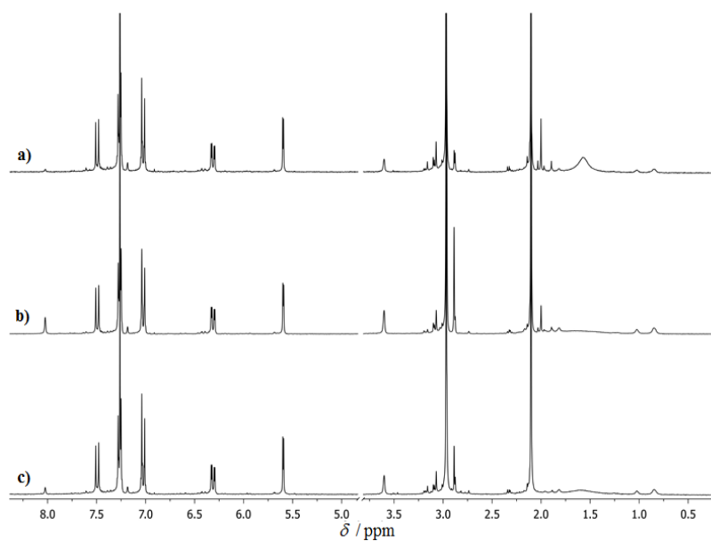
Slika 8.24: ^1\text{H} -NMR spektri produkta M2-IIa dobivenog mljevenjem L2 s [\text{Pd}(\text{OAc})_2]_3 u množinskom omjeru 3:1 uz dodatak DMF-a nakon a) 7 h (prisutna forma III ), b) nakon 12 h (prisutna forma I ) i c) nakon 20 h (prisutna forma II ). Spektri su snimljeni u \text{CDCl}_3 :
