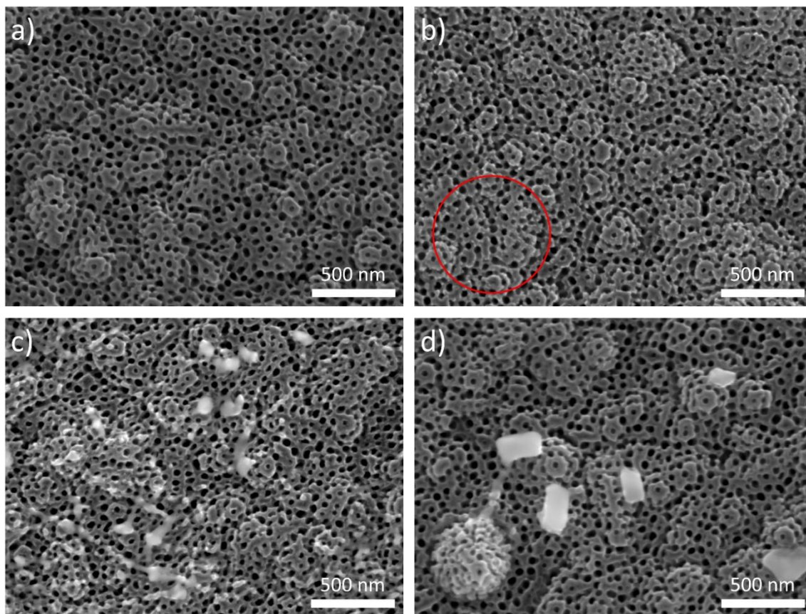
Slika 85. FE-SEM mikrografi a) TNC, te modificiranih TNC rotacijskim oblaganjem otopinama b) 12,5 mM, c) 25 mM i d) 50 mM Ba(OH) 2 .
