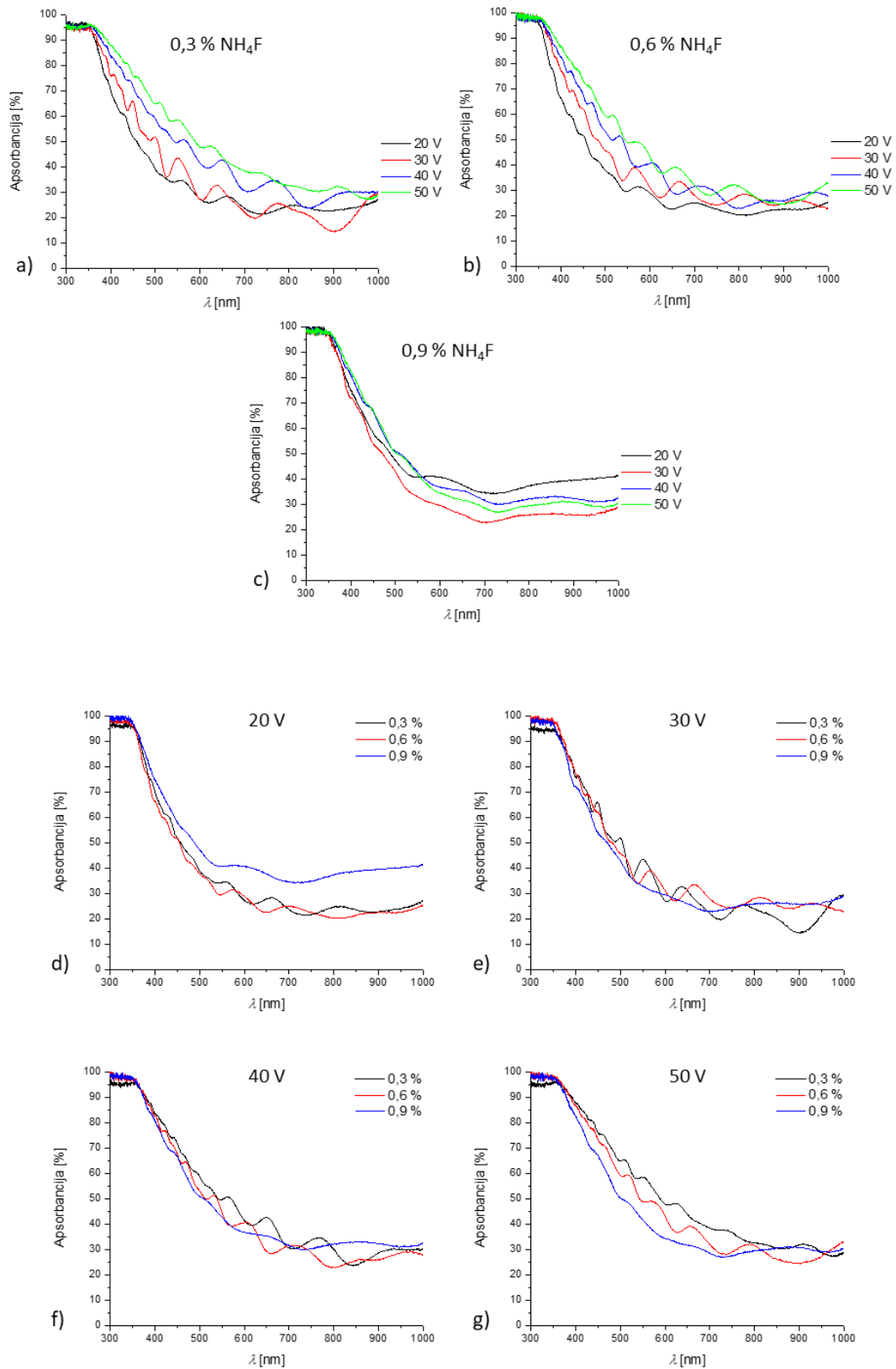
Slika 76. Optička svojstva (apsorbancija) TNC dobivenih anodizacijom tankih filmova Ti koristeći različite napone i udjele NH 4 F. Radi usporedbe prikazani su grupirana mjerenja uzoraka pri rasponima napona u odnosu na a) 0,3, b) 0,6 i c) 0,9 % NH 4 F elektrolitu i rasponima koncentracija u odnosu na napone d) 20, e) 30, f) 40 i g) 50 V.
