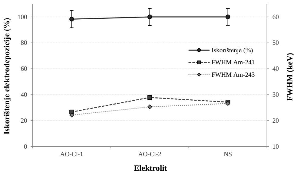
Slika 4.6. Prikaz ovisnosti iskorištenja elektrodepozicije ^{241}\text{Am} i ^{243}\text{Am} (uz standardne proširene mjerne nesigurnosti, k = 2 ) na katodi od nehrđajućeg čelika o koncentraciji i vrsti elektrolita sastava (\text{NH}_4)_2\text{C}_2\text{O}_4/\text{HCl} te \text{Na}_2\text{SO}_4 , uz odgovarajuće širine pikova (FWHM) u alfa-spektrima
