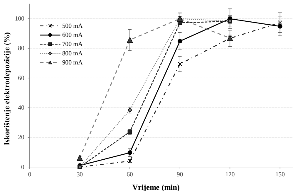
Slika 4.15 Prikaz ovisnosti iskorištenja elektrodepozicije ^{241}\text{Am} i ^{243}\text{Am} na katodi od nehrđajućeg čelika o vremenu trajanja elektrolize za različite jakosti struja u elektrolitu sastava AO-Cl-1
