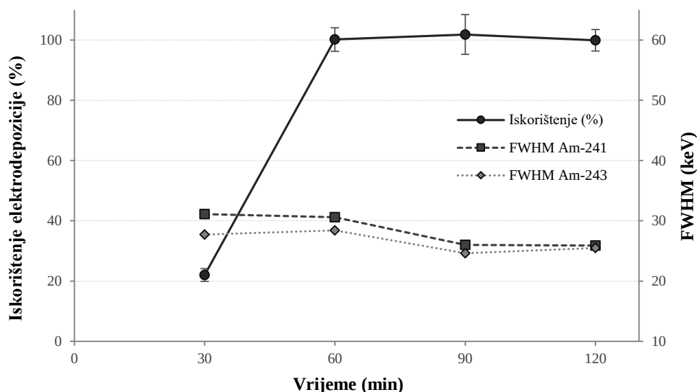
Slika 4.26. Prikaz ovisnosti iskorištenja elektrodepozicije ^{241}\text{Am} i ^{243}\text{Am} (uz standardne proširene mjerne nesigurnosti, k = 2 ) na bakrenoj katodi o vremenu trajanja elektrolize, uz odgovarajuće širine pikova (FWHM) u alfa-spektrima za NS elektrolit
