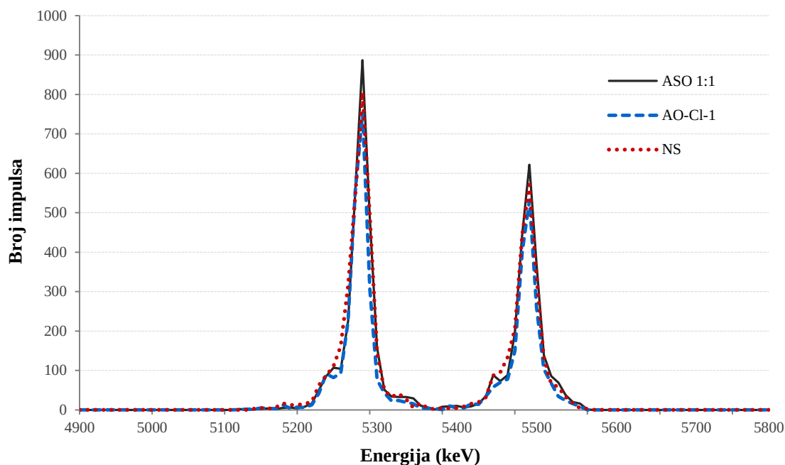
Slika 4.9. Prikaz alfa-spektara izvora ^{241}\text{Am} i ^{243}\text{Am} pripremljenih elektrodpozicijom na katodi od nehrđajućeg čelika iz otopina elektrolita sastava ASO 1:1, AO-Cl-1 i NS
