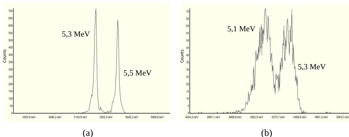
Slika 4.38. Prikaz alfa-spektara izvora ^{241}\text{Am} i ^{243}\text{Am} pripremljenih elektrodepozicijom na bakrenoj katodi, tretiranih po završetku elektrodepozicije na temperaturi (a) 500 °C i (b) ~ 1800 °C
