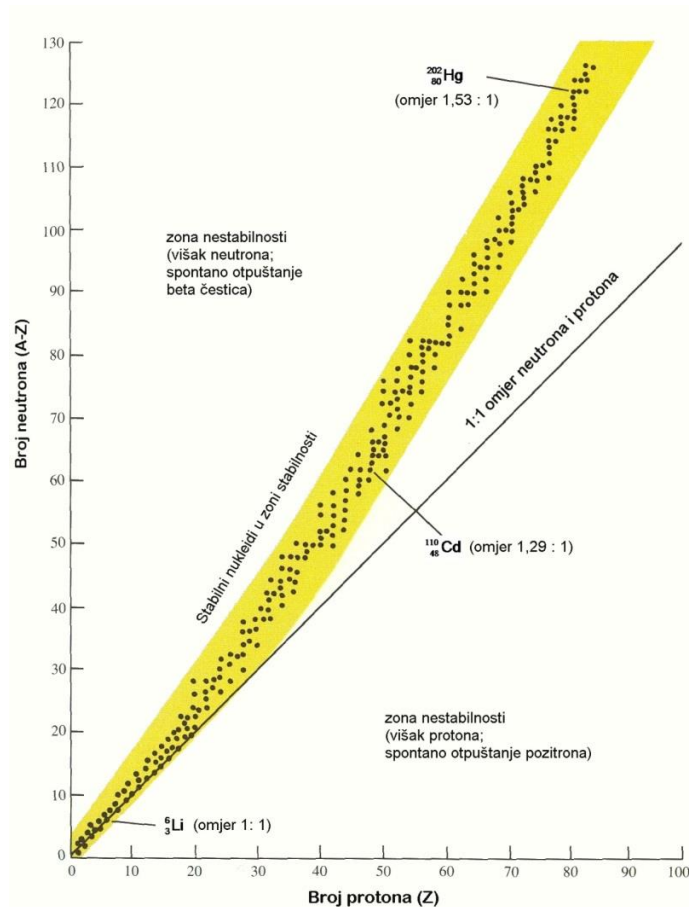
Slika 2.1. N - P dijagram zone stabilnosti jezgara (stabilni nuklidi označeni su crnim točkama) 70
