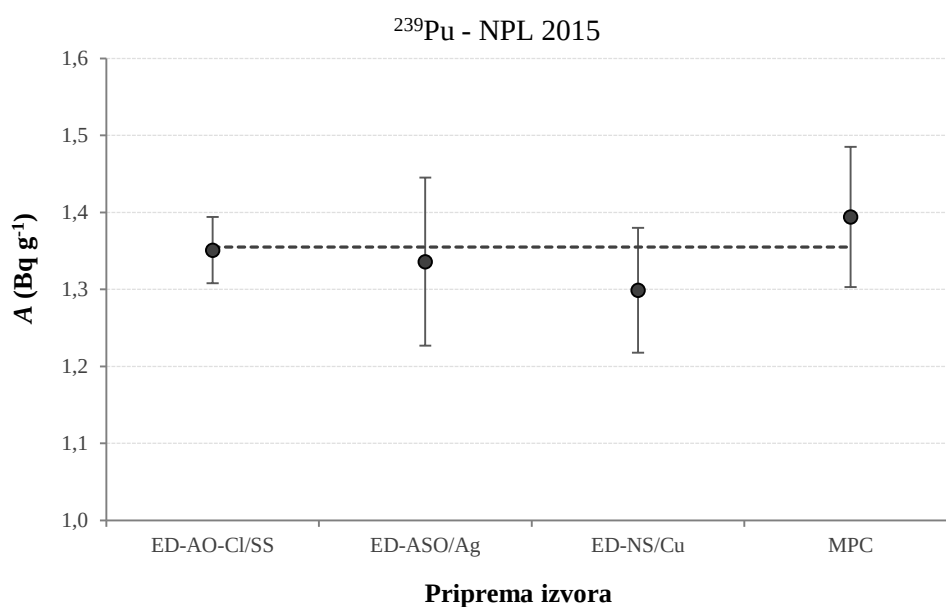
Slika 4.40. Masene aktivnosti ^{239}\text{Pu} (uz standardne proširene mjerne nesigurnosti, k = 2 ) u NPL 2015 uzorku (alfa-izvori pripremljeni metodom mikro-koprecipitacije i elektrodpozicije pri optimiranim uvjetima)
