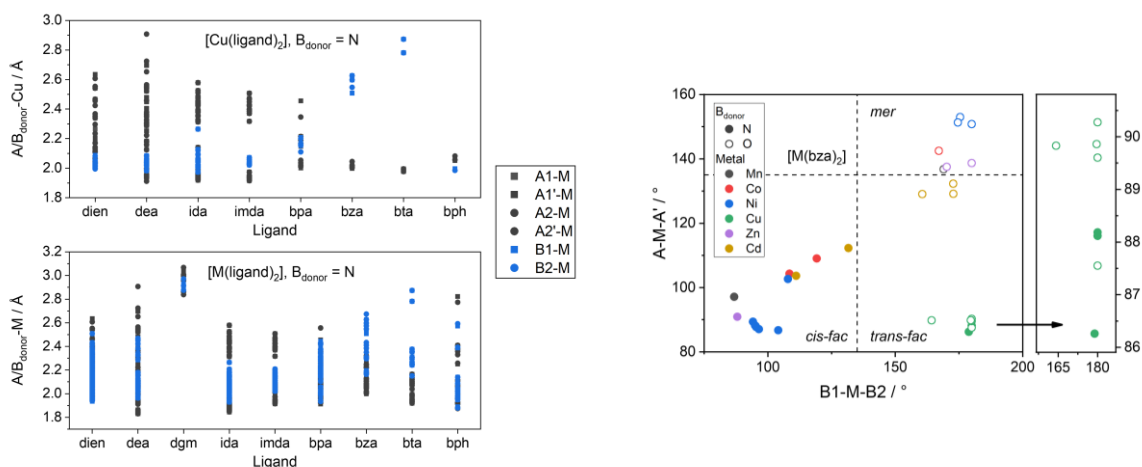
Slika 19. Duljine A/B donor -M veza za ligande s B donor = N, za Cu(II) komplekse i sve analizirane komplekse (lijevo). Ovisnost A-M-A' o B1-M-B2 kutovima za 16 N-bza i 15 O-bza liganada (desno).
