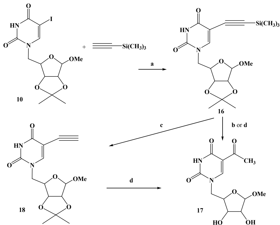
Scheme 2. (a) \text{PdCl}_2(\text{PPh}_3)_2 , CuI, \text{Et}_3\text{N} ; (b) Amberlite IR-120 ( \text{H}^+ ), MeOH, reflux; (c) NaOMe/MeOH, rt; (d) 50 % TFA/ \text{H}_2\text{O} .
